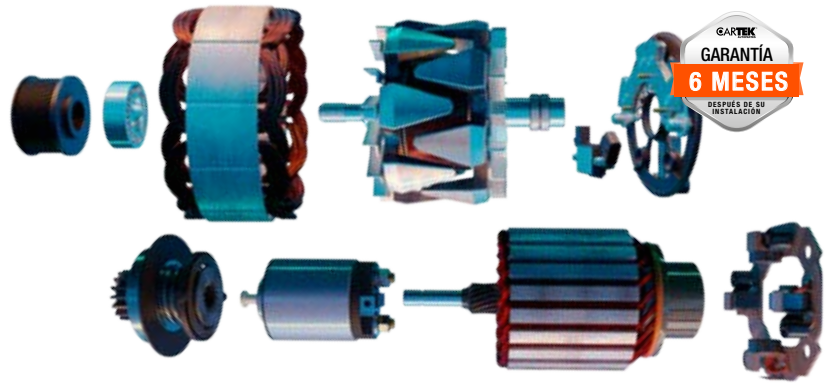
• Polea • Estator • Rotor • Portacarbon • Carbon • Impulsor • Armadura • Solenoide 48
